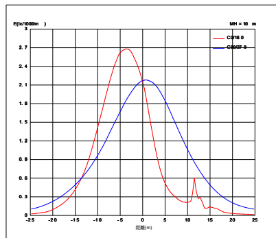
照度曲線
