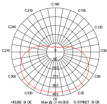
光度分布図
