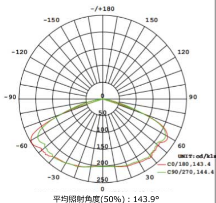
発光強度分布図
