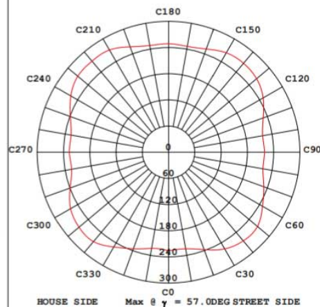
最大強度表面分布図
